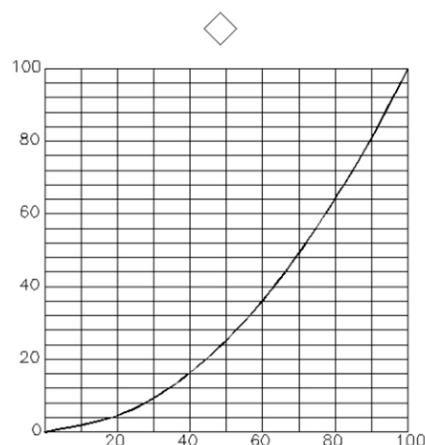
VERTICAL: % MAXIMO DE CAUDAL HORIZONTAL: % DE APERTURA DE LA VALV. (diafragma cuadrangular)
